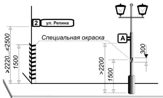
Рисунок 75 – Особенности размещения и параметры визуальных указателей в пределах пешеходного пути
