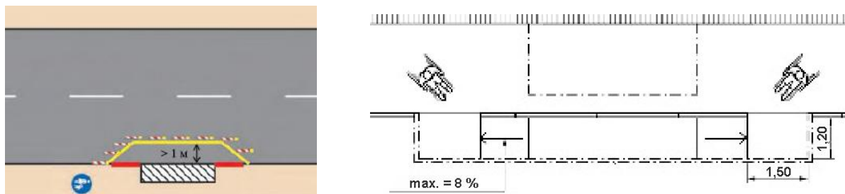
Рисунок 58 – Примеры обустройства временного пешеходного пути
