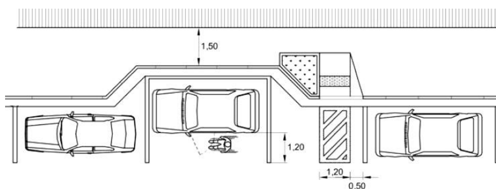
Рисунок Б.3 – Типовая схема планировки машино-места для стоянки (парковки) транспортного средства инвалида в заездном «кармане» параллельно тротуару
