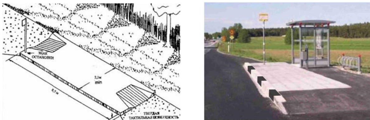
Рисунок 48 – Пример обустройства остановочного пункта пандусами
