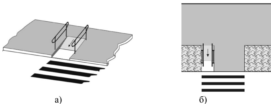
Рисунок 25 – Вариант размещения пандусов на отнесенных пешеходных переходах и пешеходных переходах, располагаемых на перегонах
