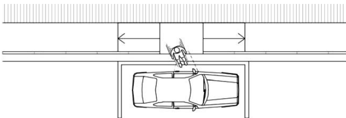
Рисунок Б.5 – Типовая схема планировки машино-места для стоянки (парковки) транспортного средства инвалида параллельно тротуару на левой стороне проезжей части автомобильной дороги с односторонним движением для стесненных условий
