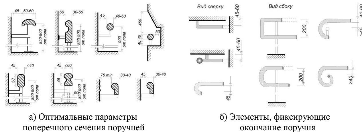
Рисунок 13 – Основные параметры конструкции поручней
