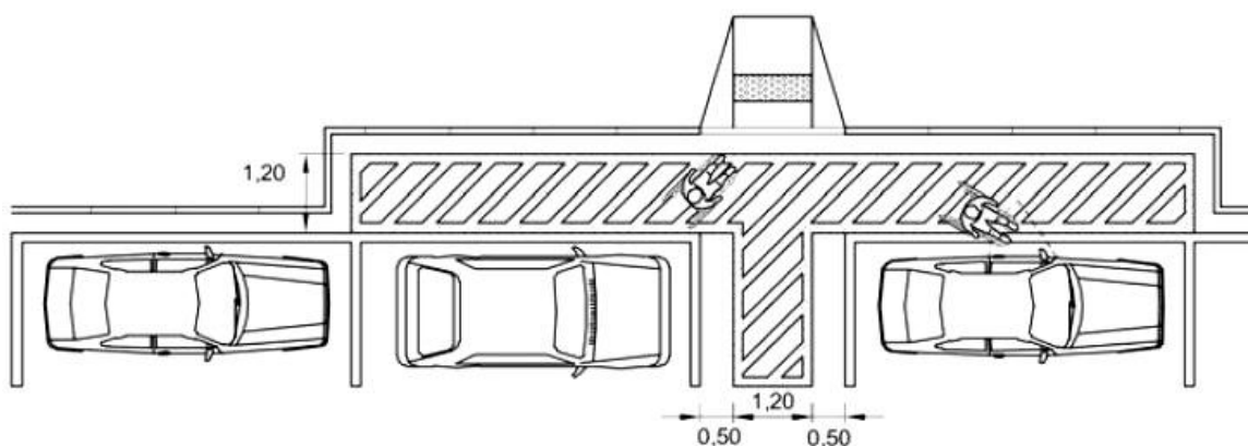
Рисунок Б.6 – Типовая схема планировки машино-места для стоянки (парковки) транспортного средства инвалида параллельно тротуару на левой стороне проезжей части автомобильной дороги с односторонним движением, оборудованной «карманом» для подхода к транспортным средствам
