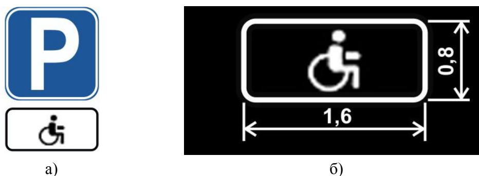
Рисунок 55 – Пример обозначения машино-места для стоянки (парковки) транспортного средства инвалидов с использованием дорожных знаков (а) и дорожной разметки (б)
