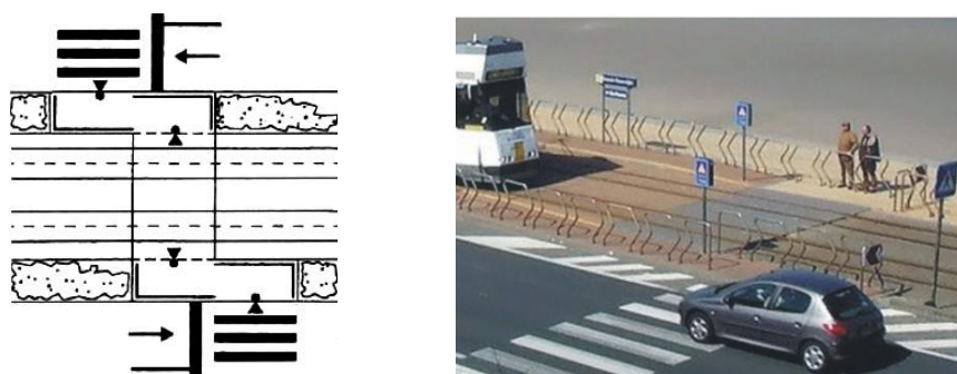
Рисунок 43 – Пример размещения пешеходного перехода через трамвайные пути
