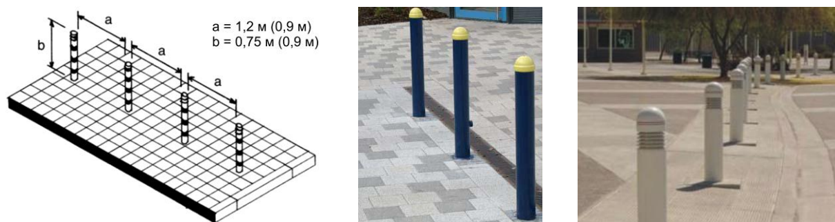
Рисунок 66 – Примеры ограждений, используемых в качестве направляющих устройств
