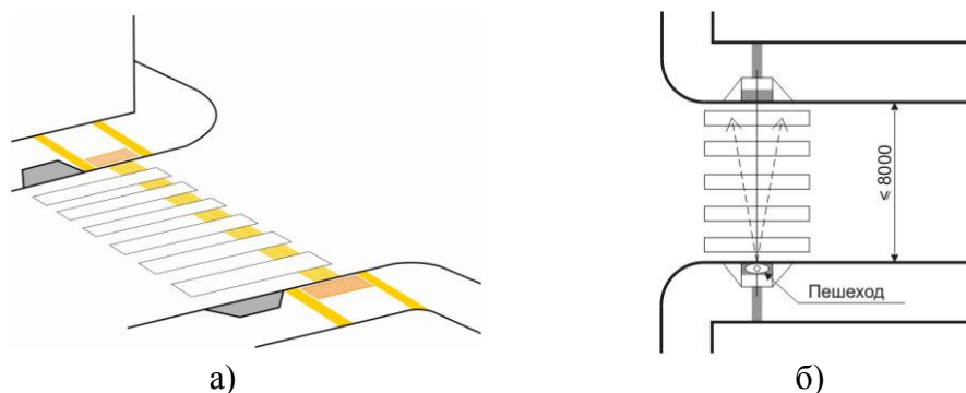
Рисунок 64 – Примеры обустройства пешеходных переходов тактильной направляющей поверхностью
