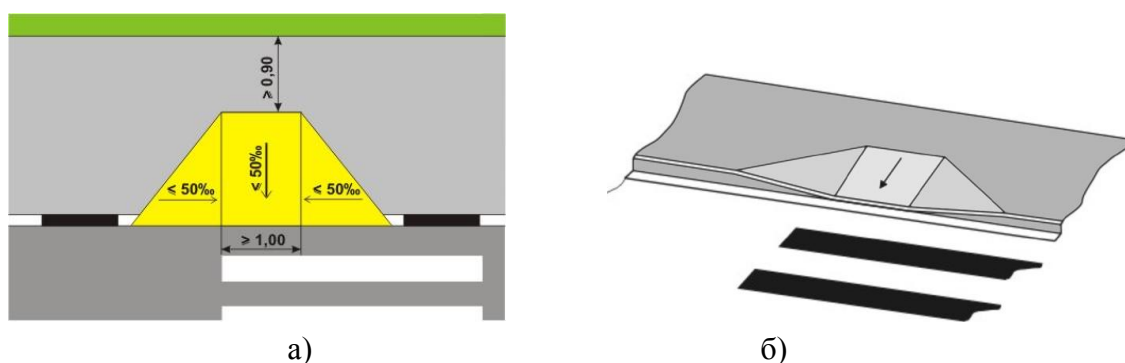
Рисунок 29 – Вариант размещения пандусов на отнесенных пешеходных переходах и пешеходных переходах, располагаемых на перегонах
