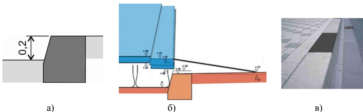
Рисунок 47 – Примеры обустройства границы посадочной и остановочной площадок, обеспечивающего доступность посадки инвалидов в транспортное средство
