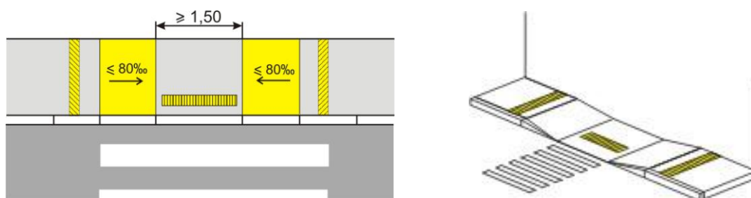
Рисунок 31 – Варианты размещения пандусов на отнесенных пешеходных переходах и пешеходных переходах, располагаемых на перегонах для стесненных условий
