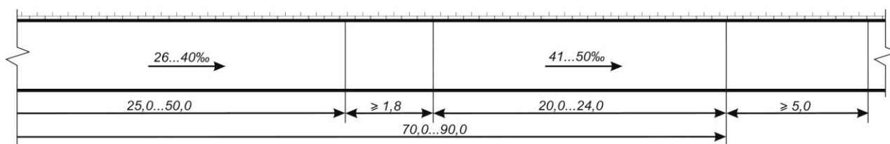
Рисунок 2 – Пример планировки тротуара (пешеходной дорожки) с продольным уклоном, соответствующим нормальным условиям движения инвалидов
