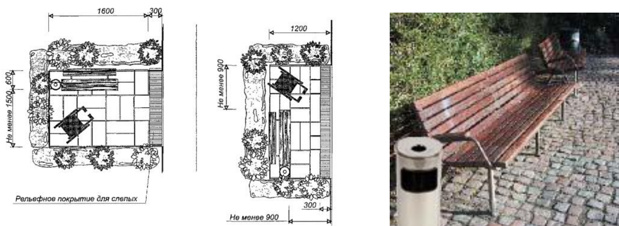
Рисунок 56 – Примеры обустройства зон отдыха инвалидов
