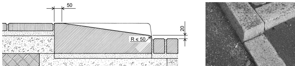
Рисунок 23 – Примеры обустройства пандуса в месте его сопряжения с проезжей частью автомобильной дороги
